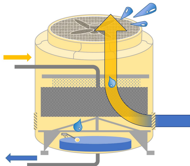
【冷却塔の模式図】
