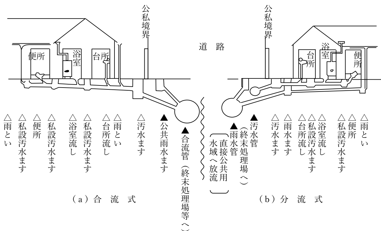
図-1 排水設備と公共下水道
