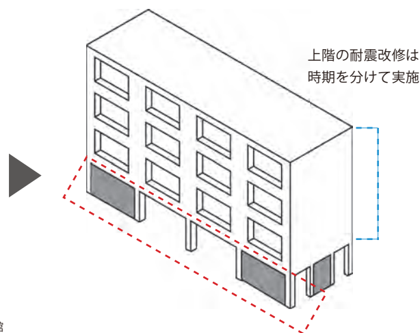
1階のピロティ部分について先行的に耐震改修を実施
