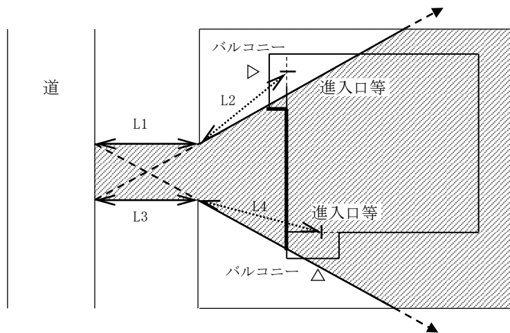
図1 「道から非常用出入口等までの延長が20m以下」及び「バルコニーのその他これらに類するものの位置」
