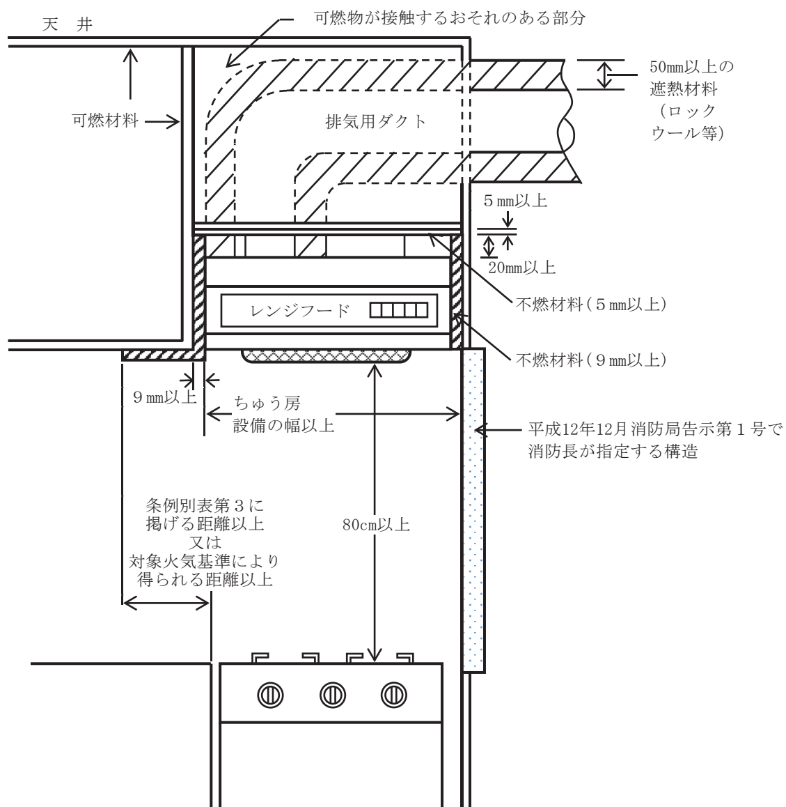
別図第5 レンジフードファンの設置例
