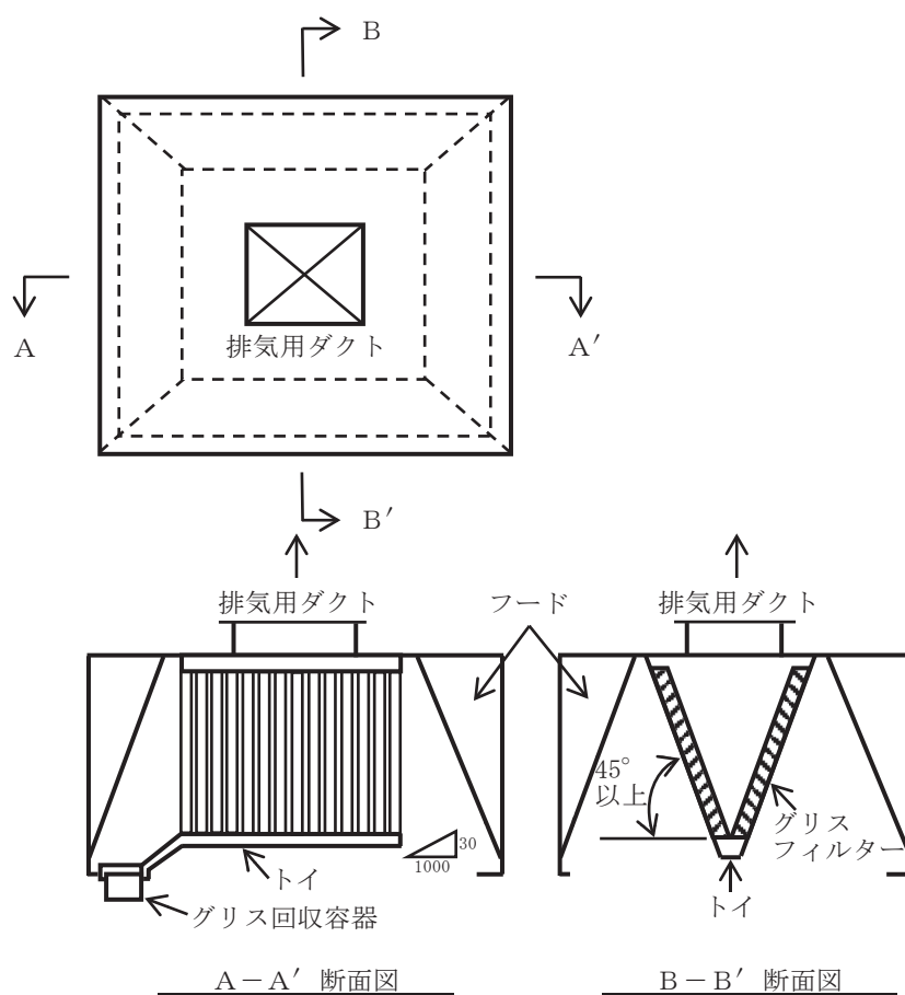
別図第3 フードの構造（排気フードI型の場合の例）
