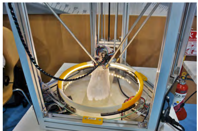
3Dプリンターによる義足製作
