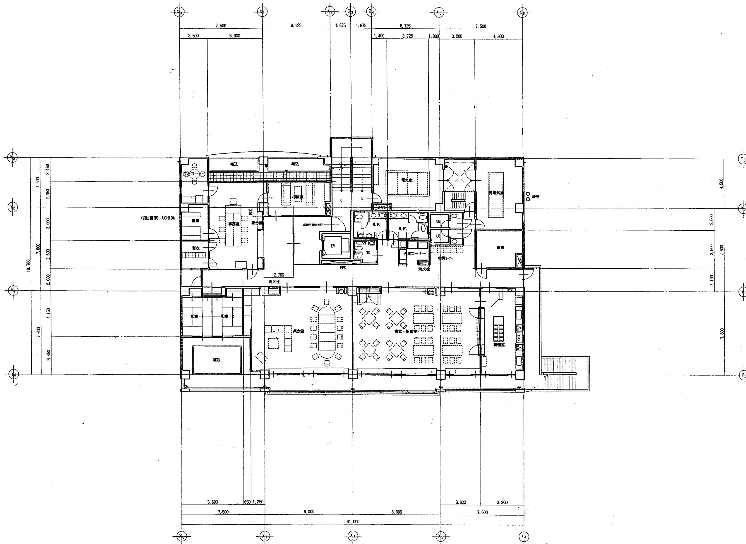
保土ヶ谷区生活支援センター 4階平面図
