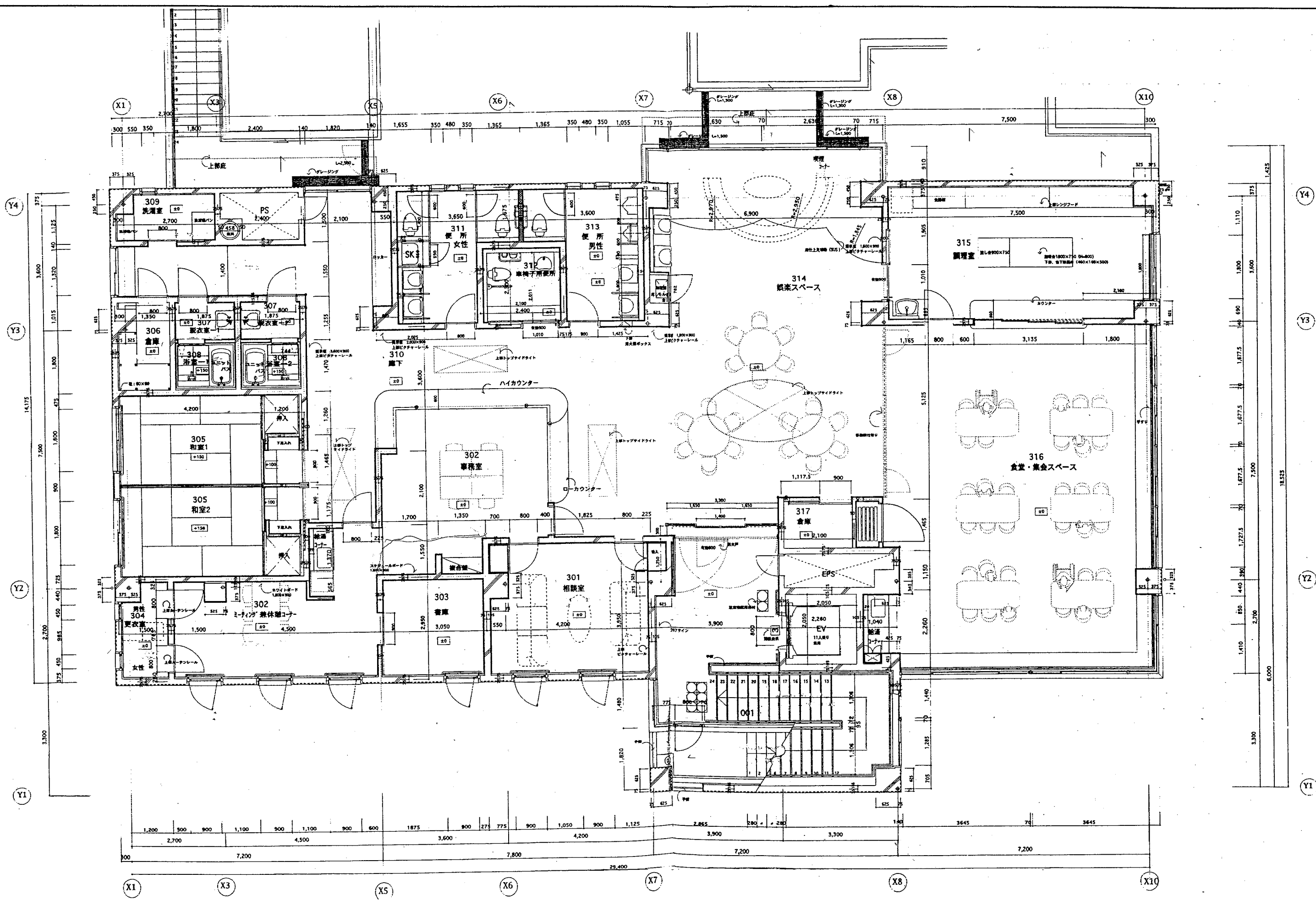
港南区生活支援センター 3階平面図
