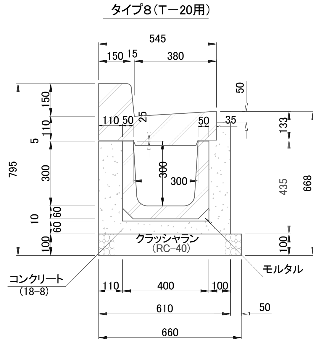
材料表
