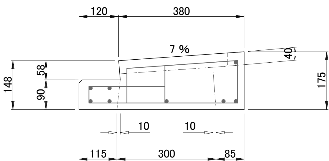
側 面 図
