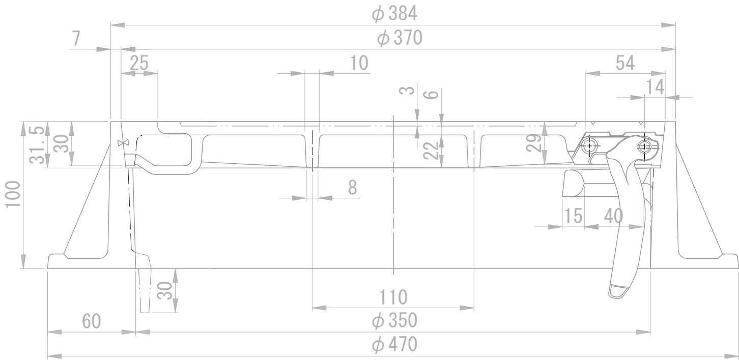
断 面
