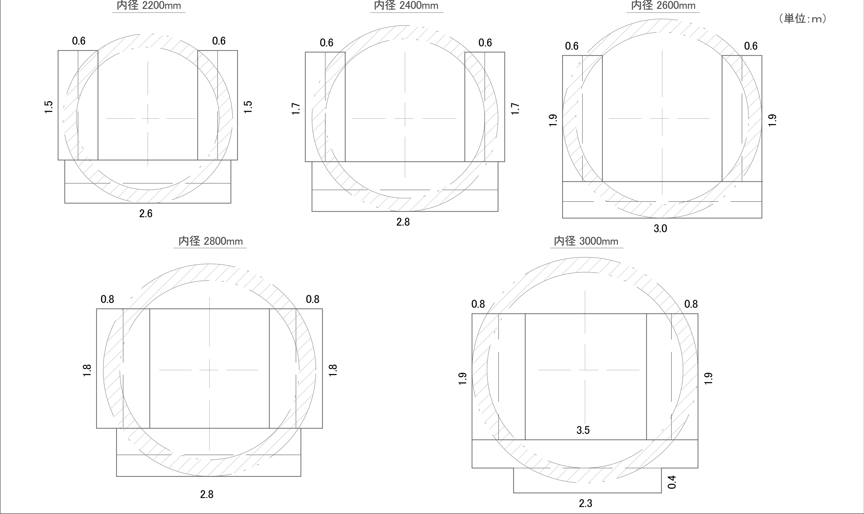
標準押角設置図(3)
