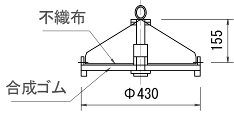
断面図
