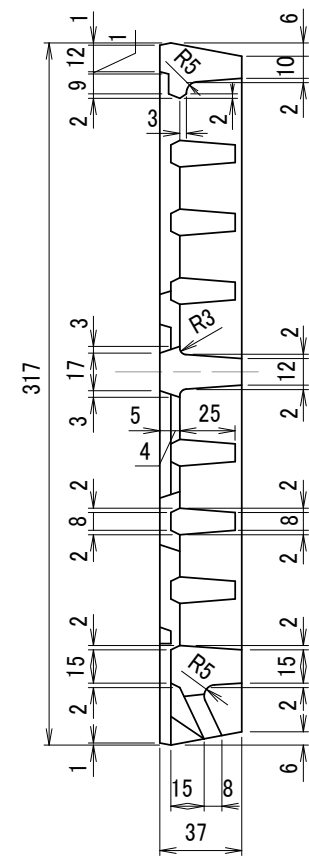
B-B断面図
