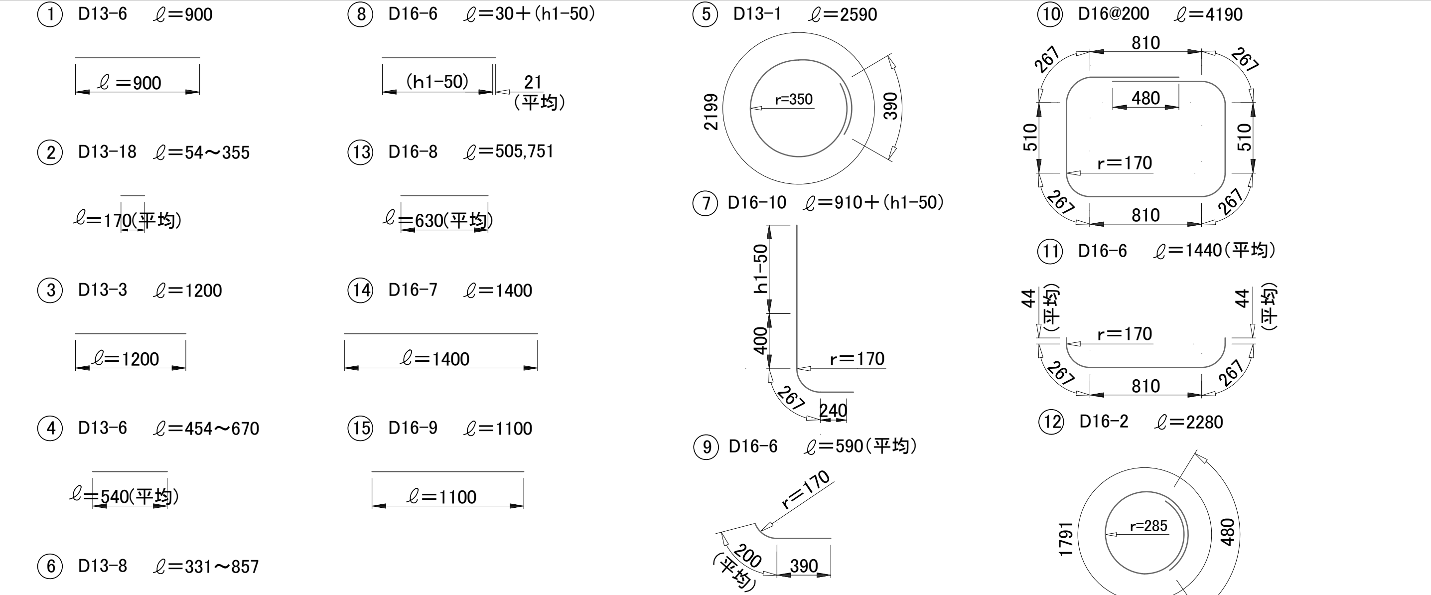
材 料 表
