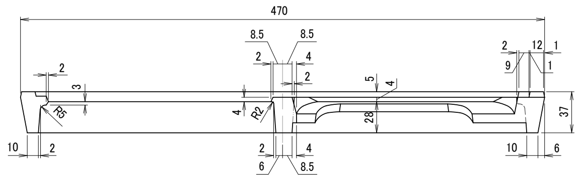
A-A断面図
