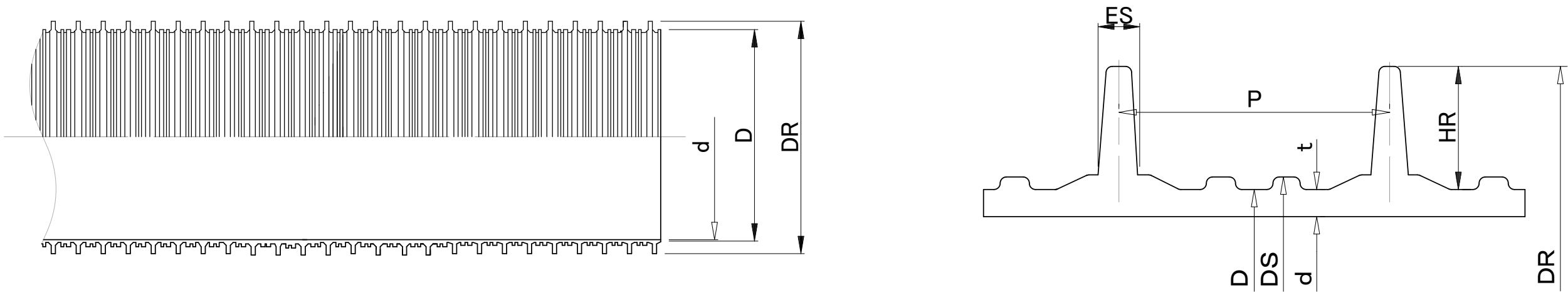
直管部共通寸法
