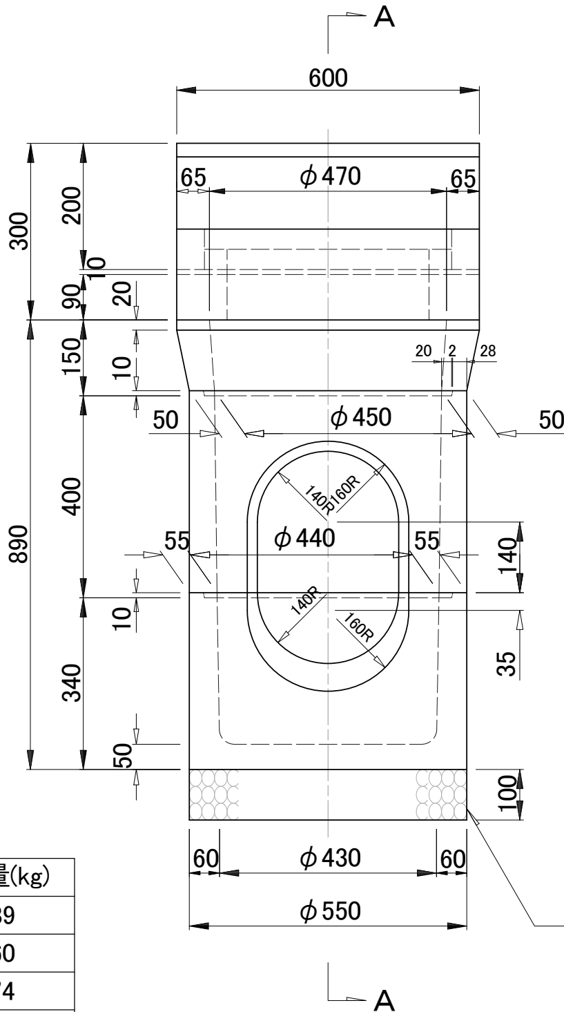
側面図
