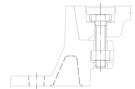
親ふたばール穴部詳細図
