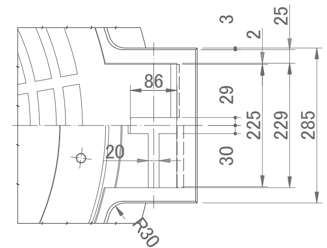
受柰蝶番取付部
