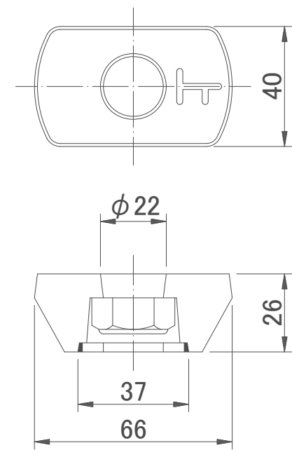
浮上り防止金具詳細図
