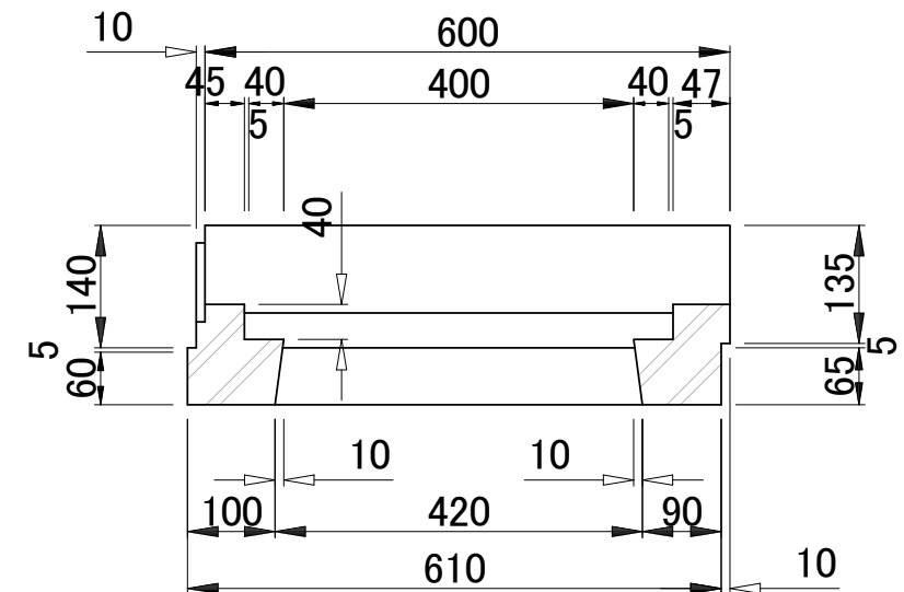
A-A 断面図
