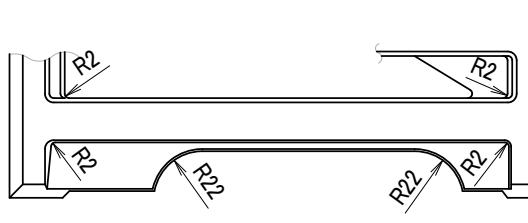
裏面図
