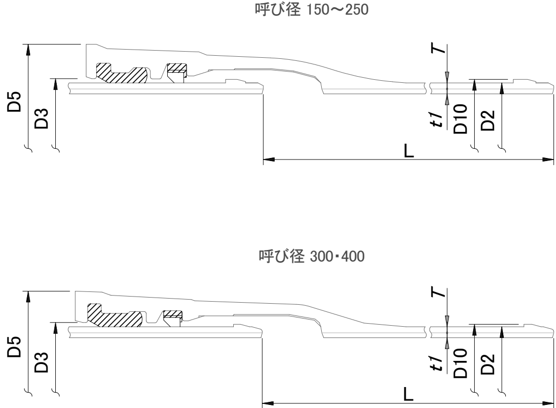
寸法表
