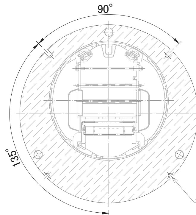
親ふた平面図
