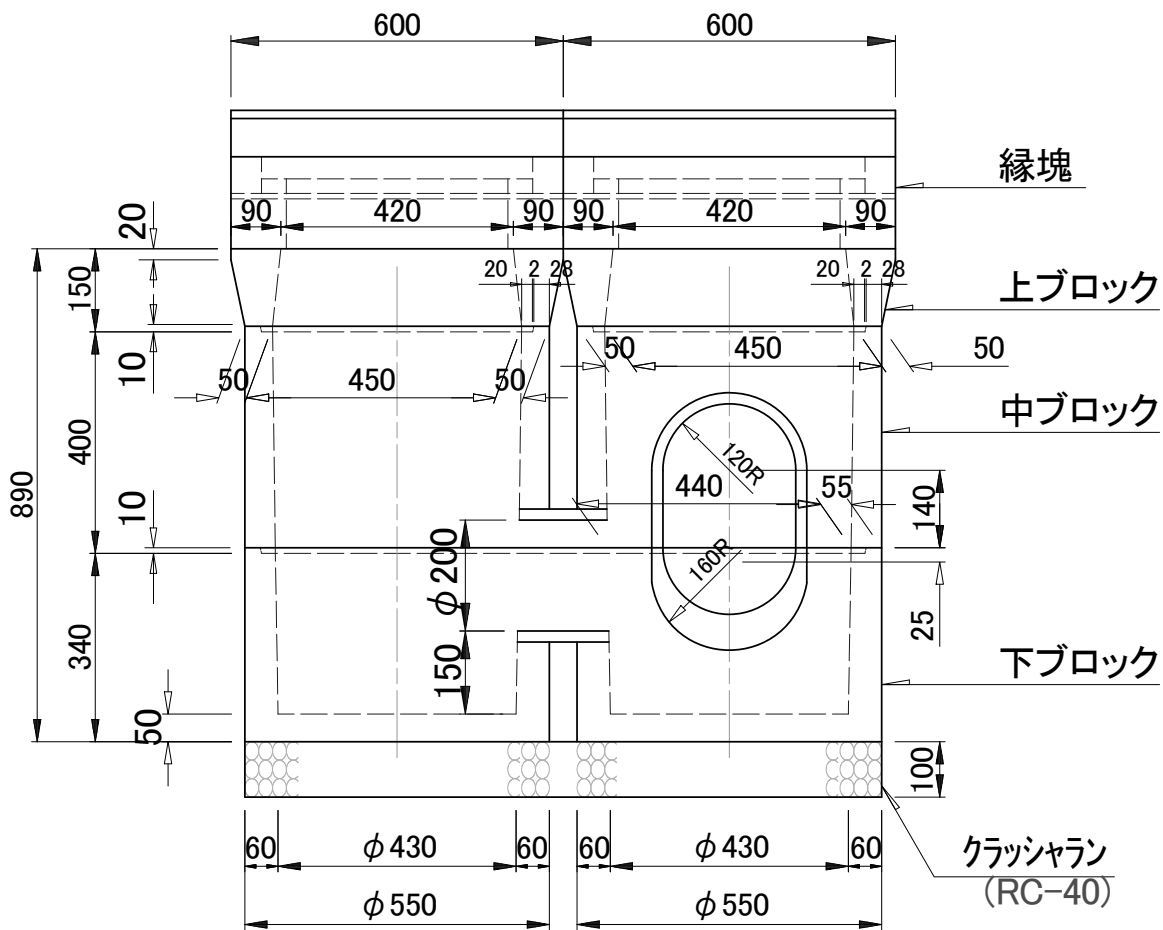
側面図
