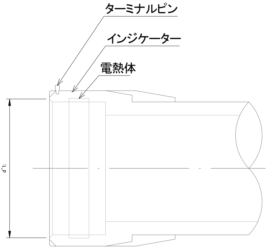
EF受口共通寸法
