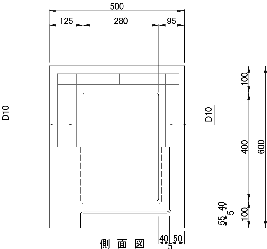
タイプ 2 用 平 面 図
