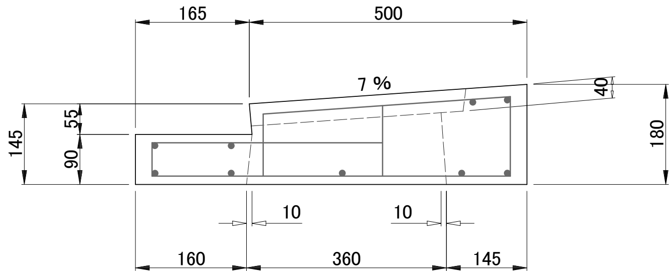
側 面 図
