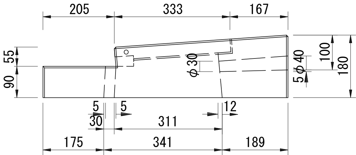
側面図
