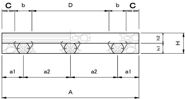
Ⓐ—Ⓐ断面
