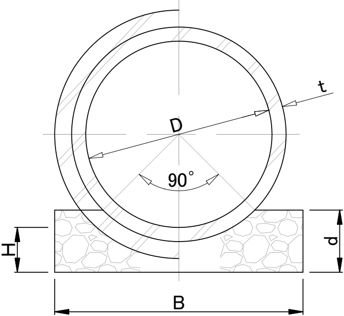
砕石 90° 基礎
