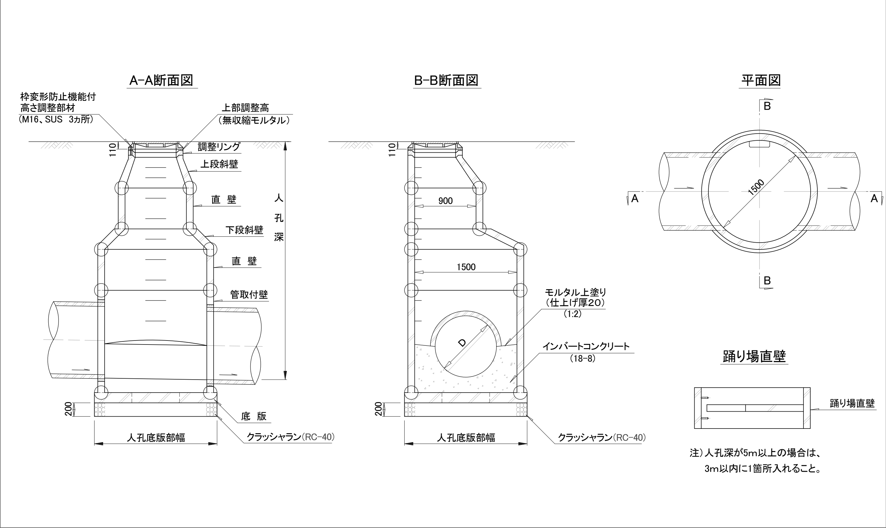
第3種組立人孔構造図 (JSWAS A-11)
