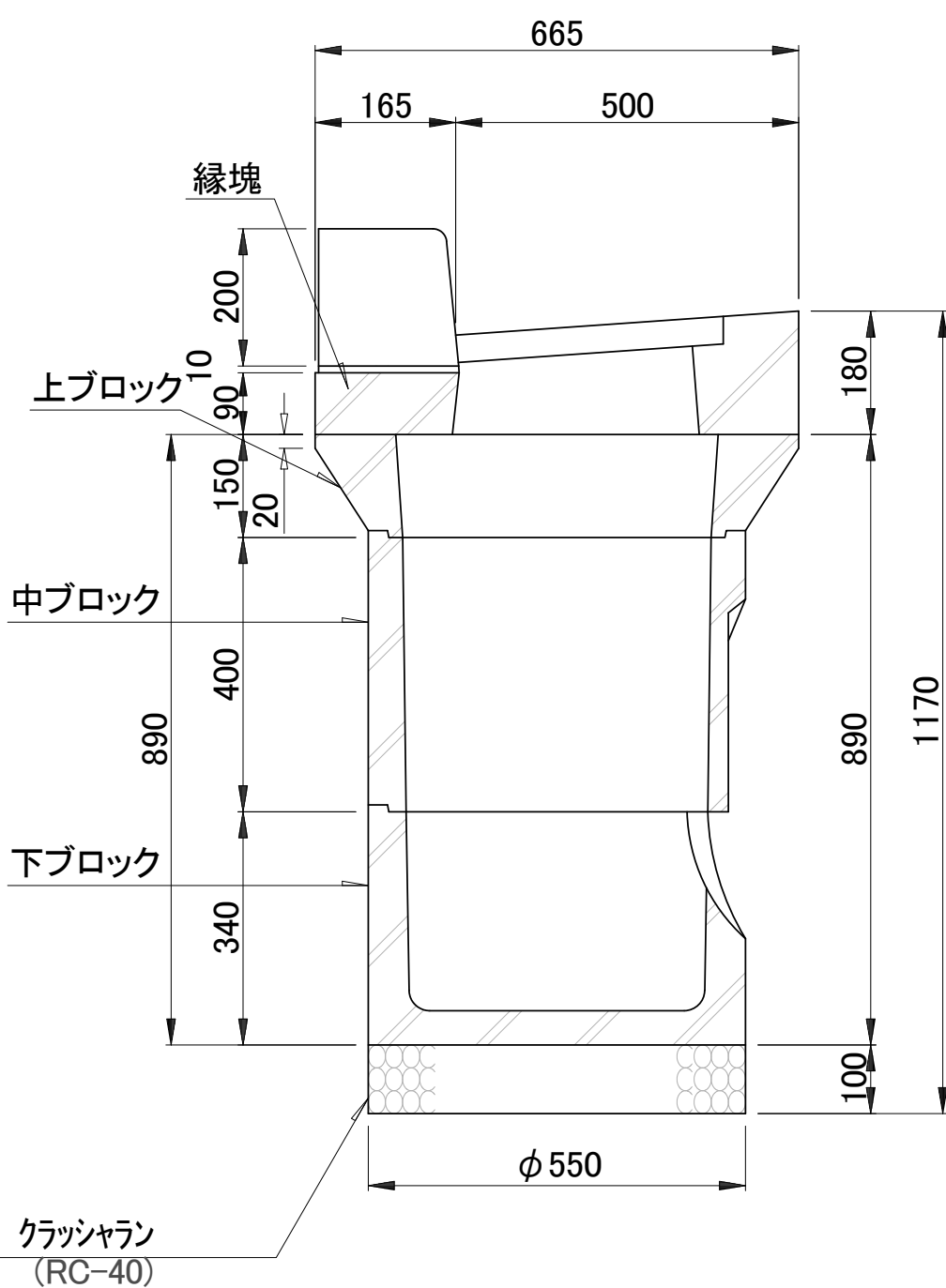
A-A断面図
