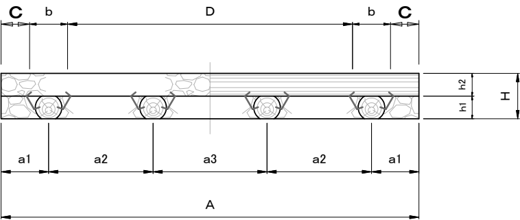
Ⓑ—Ⓑ断面
