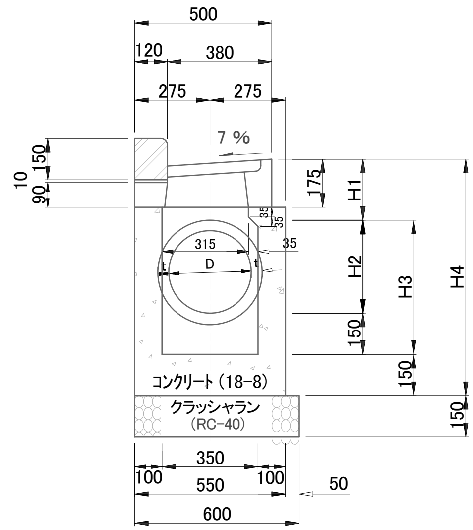
材料表及び寸法表
