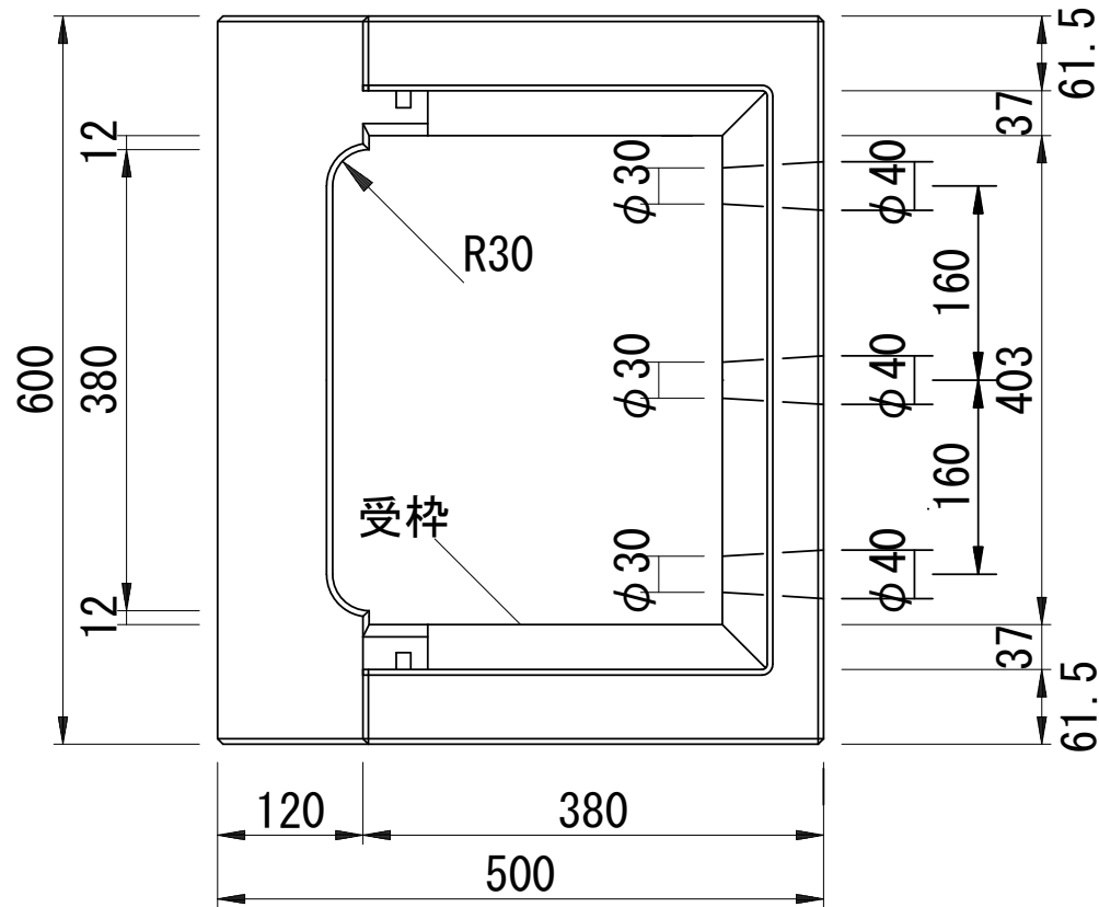
側面図
