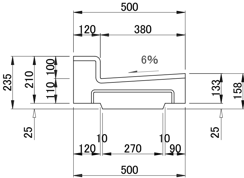
正面図
