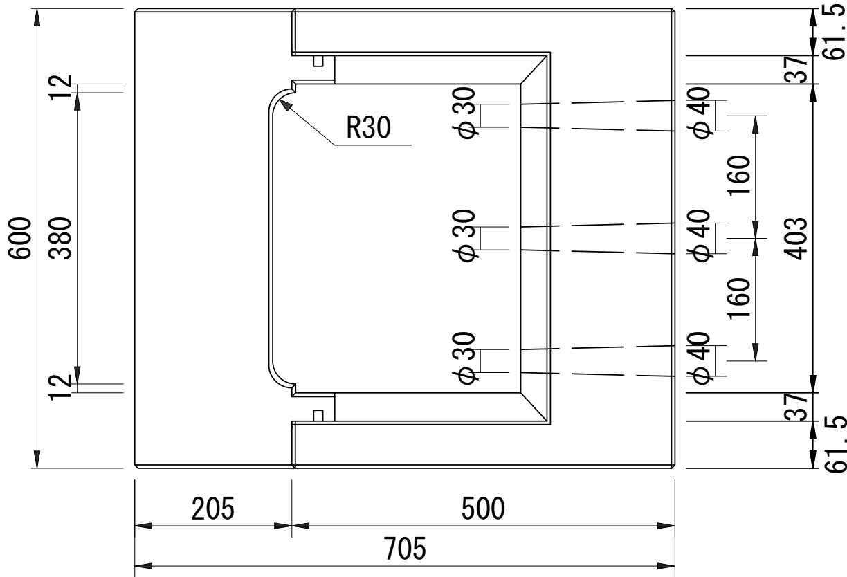
側面図
