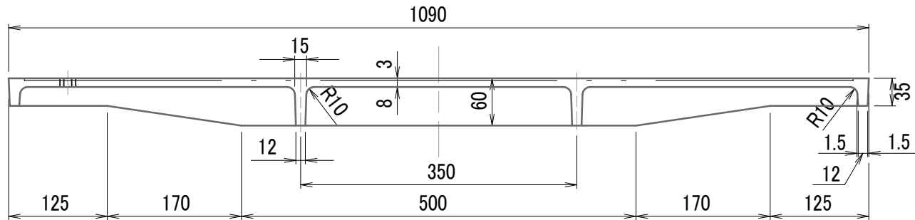
A-A断面図
