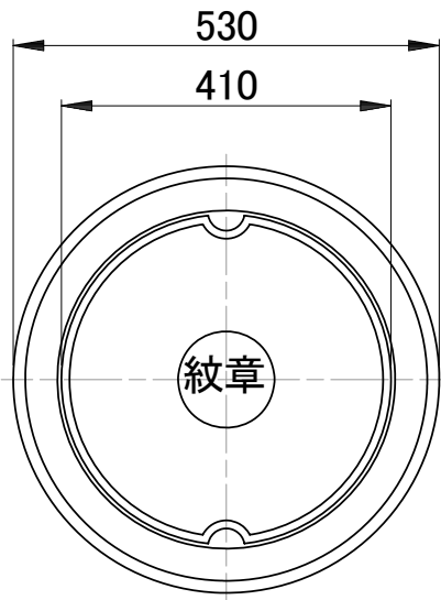
ふた 縁塊
