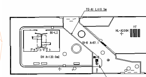
施設平面図
