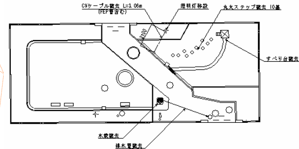
撤去・移設平面図
