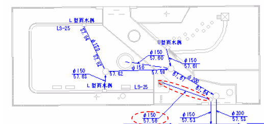
「地下埋設物(排水)」レイヤ
