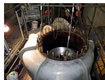
ポンプの再整備（長寿命化）
