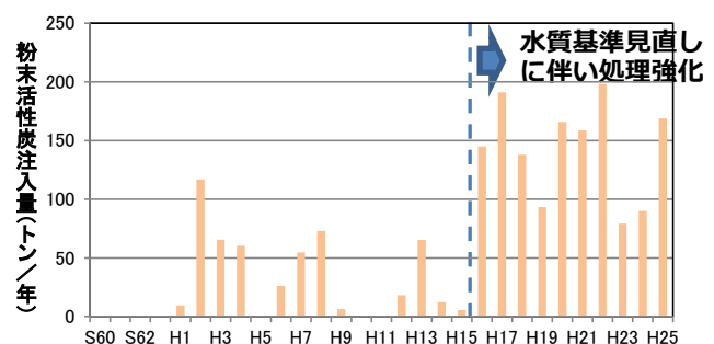
西谷浄水場における活性炭の使用量
