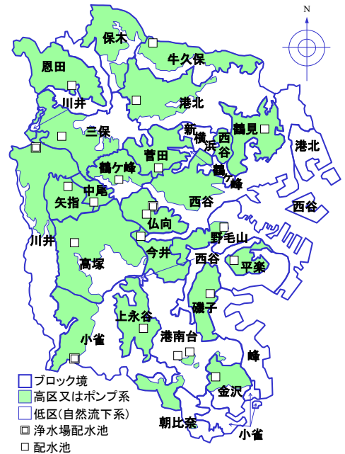
配水ブロックシステム
