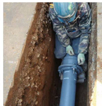
耐震管の布設状況
