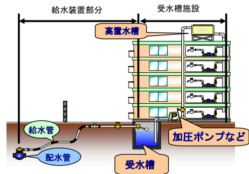
給水装置と受水槽施設の範囲
