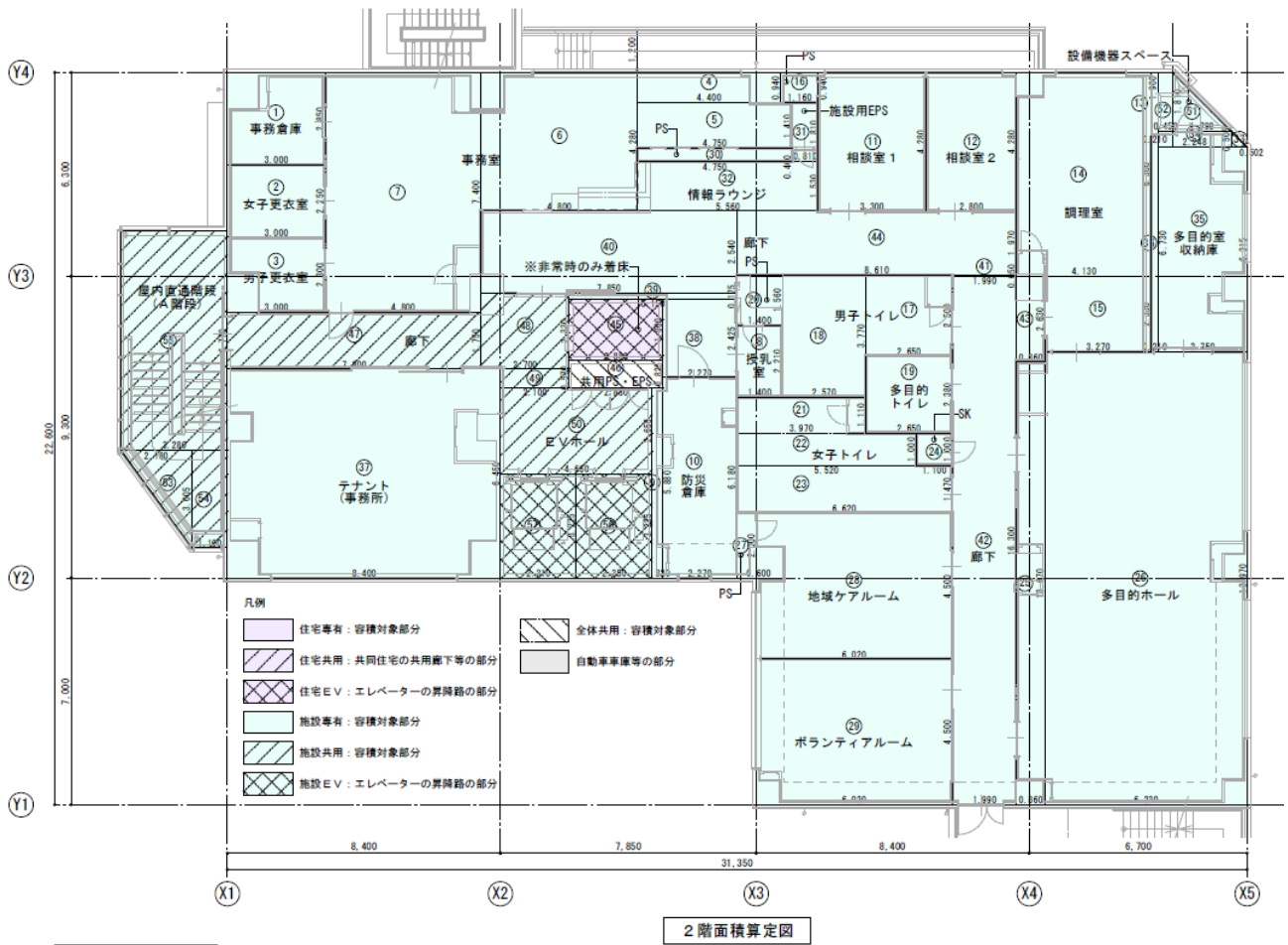
2 階面積算定図
