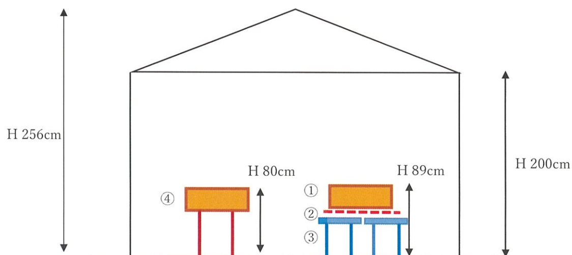
<立面図>
