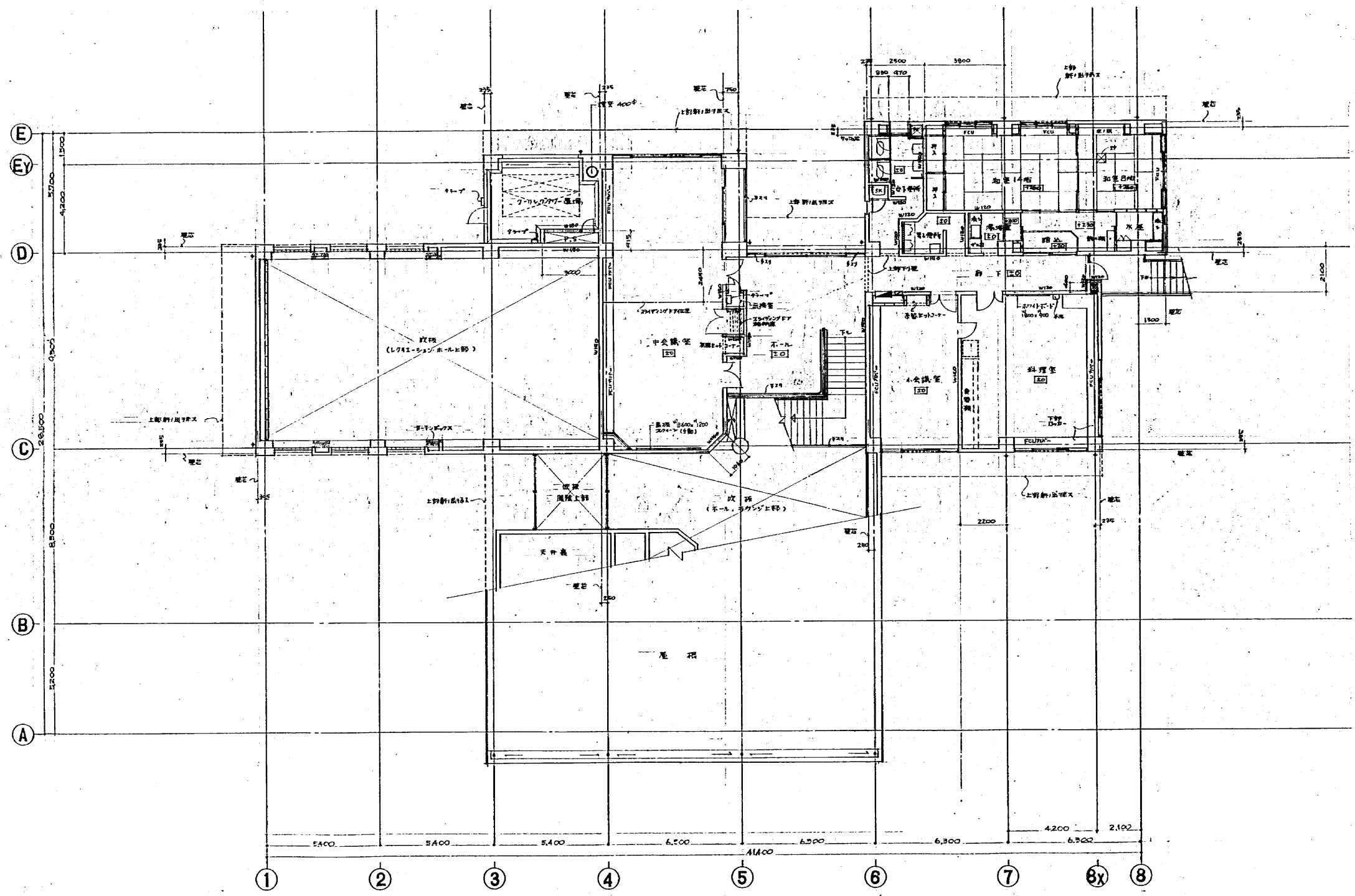
2階平面図 1/100
