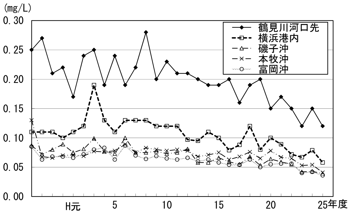
図 2-15 東京湾IV類型全隣年平均値の経年変化（公共用水域水質測定）
