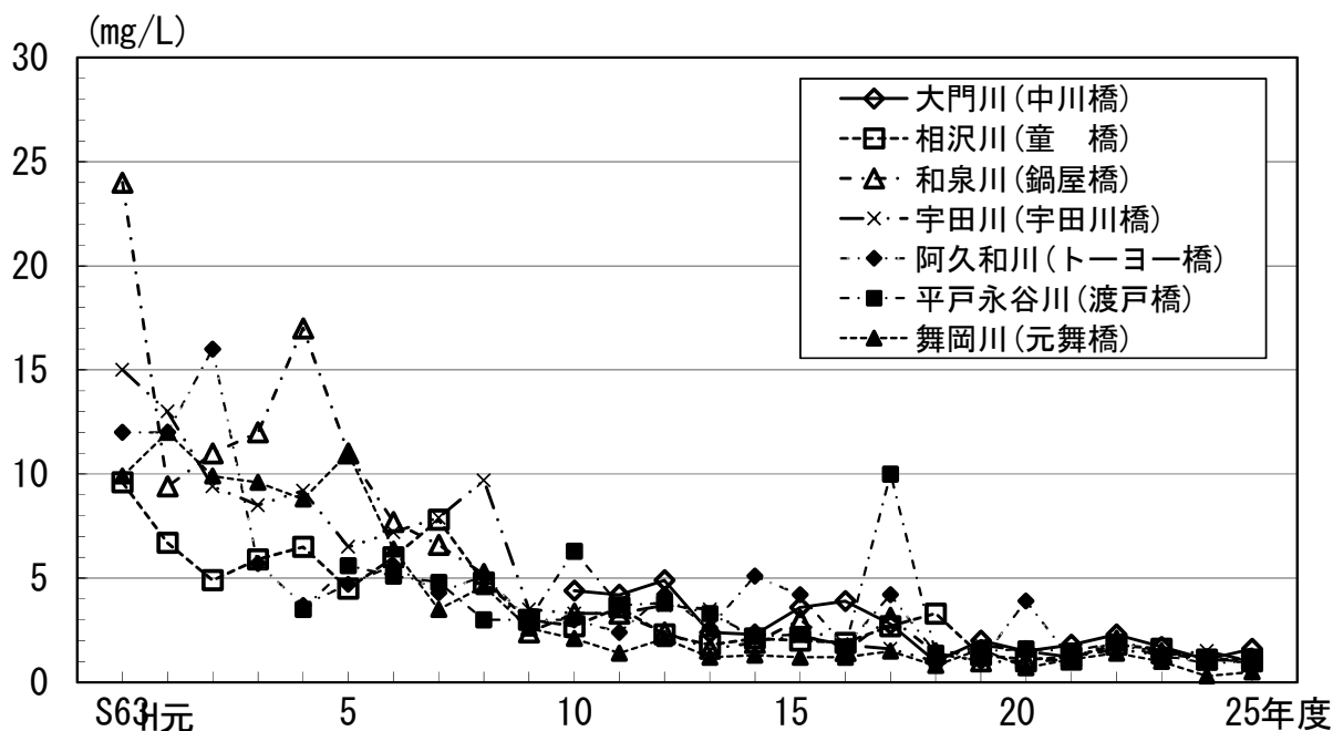
図 2-10 境川支川 BOD 年平均値の経年変化 (中小河川水質調査)
