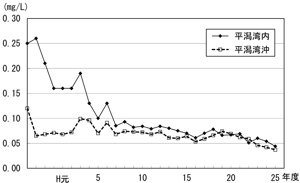
図 2-16 東京湾III類型全隣年平均値の経年変化（公共用水域水質測定）
