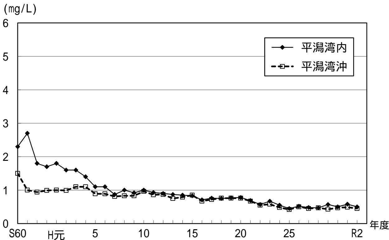
図 2 - 1 2 東京湾 類型全室素年平均値の経年変化
