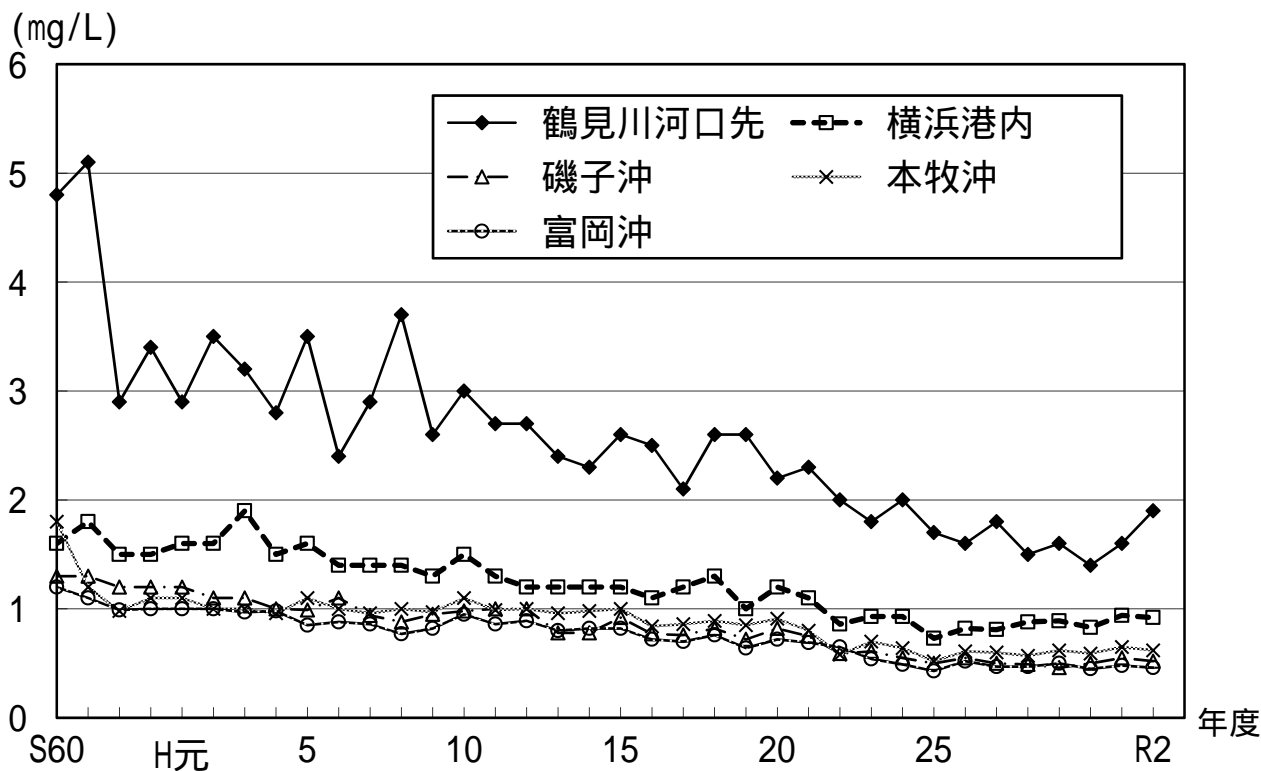
図 2 - 1 1 東京湾 類型全室素年平均値の経年変化
