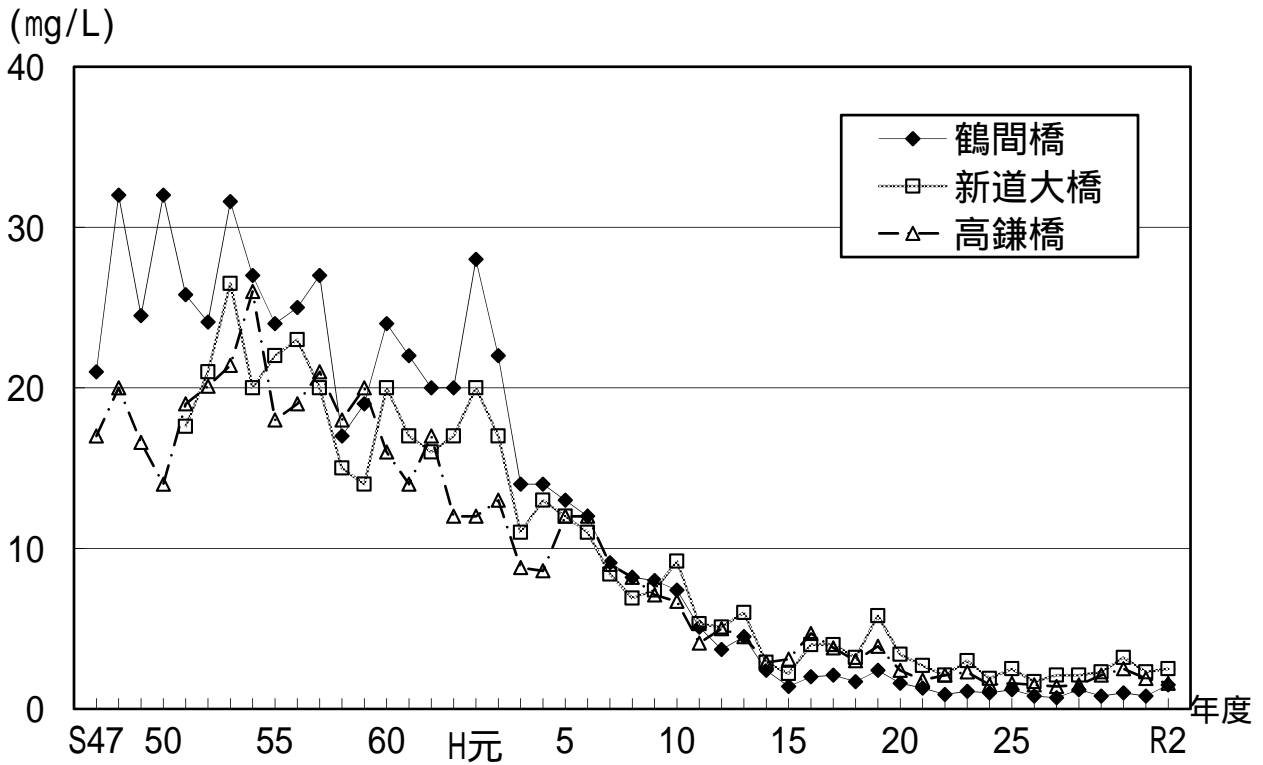
図 2 - 7 境川本川 BOD 年平均値の経年変化
