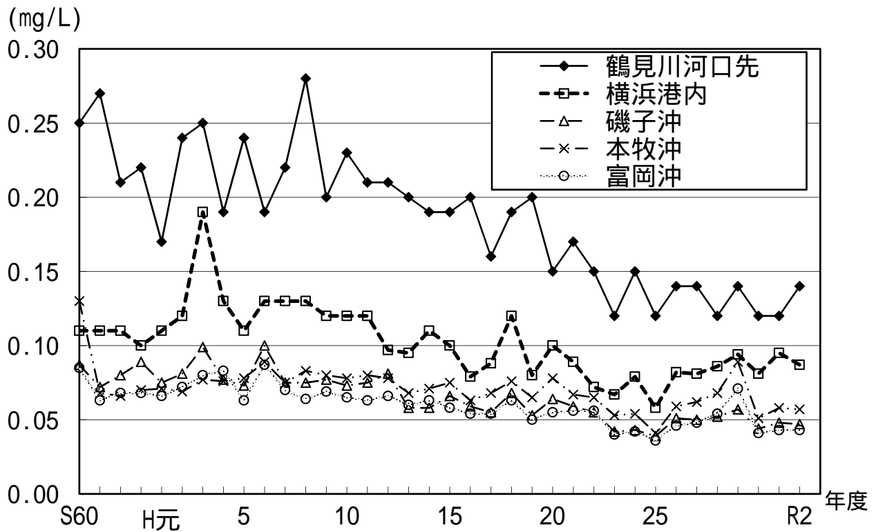
図 2 - 1 3 東京湾 類型全燐年平均値の経年変化
