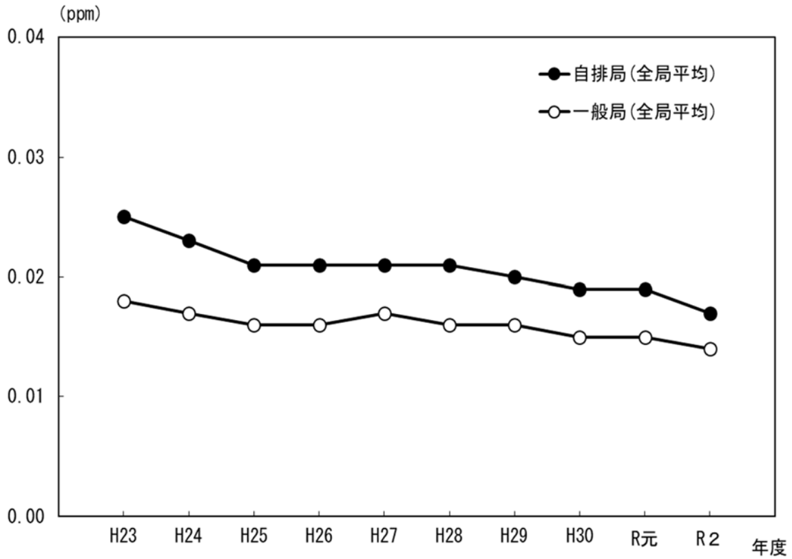
図 1 - 1 0 二酸化窒素の年平均値の経年変化
