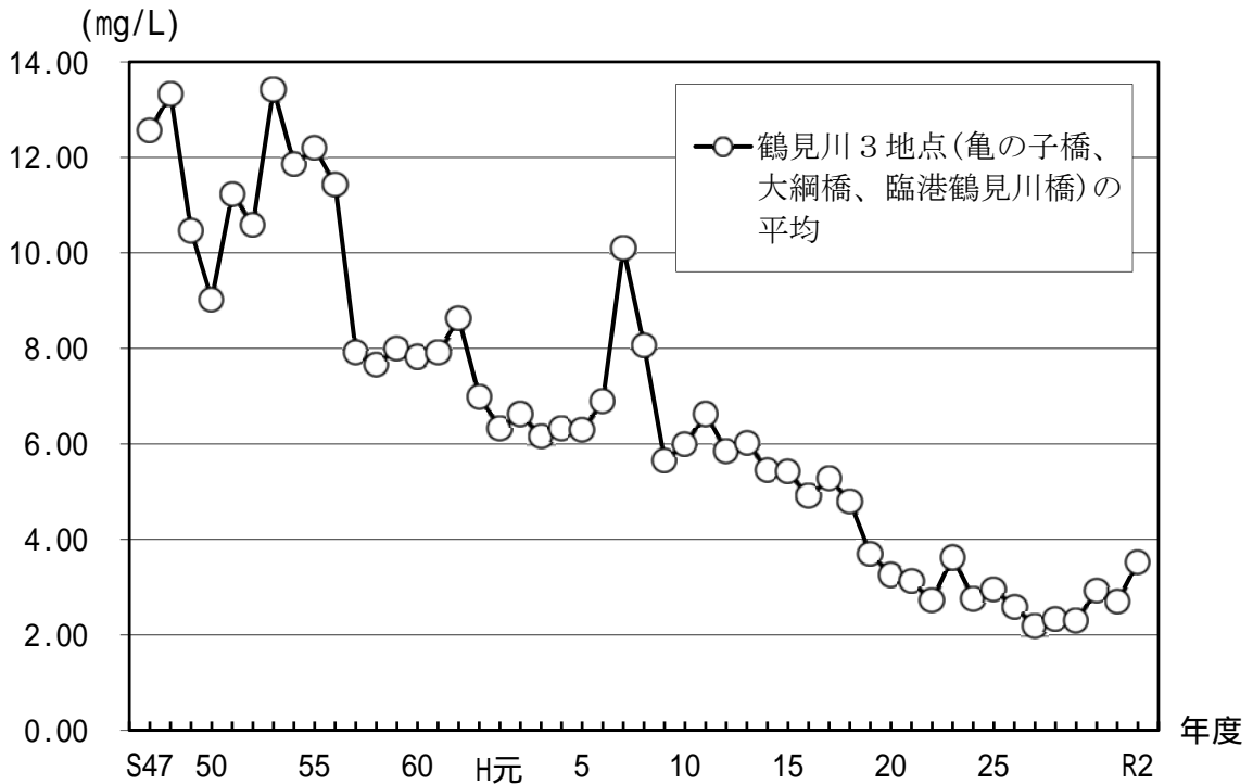
図 2 - 1 鶴見川の BOD 経年変化
