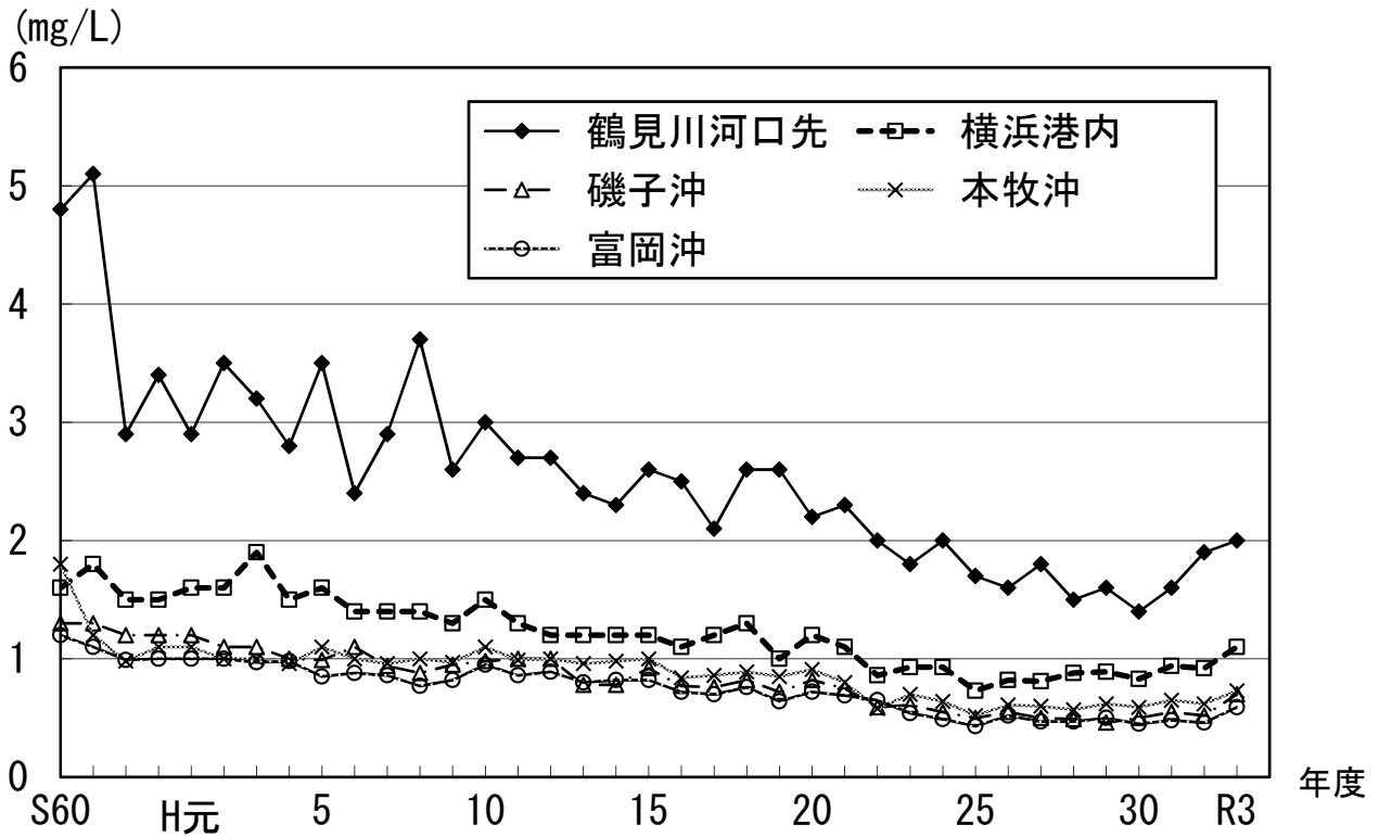
図 2-11 東京湾IV類型全窒素年平均値の経年変化
