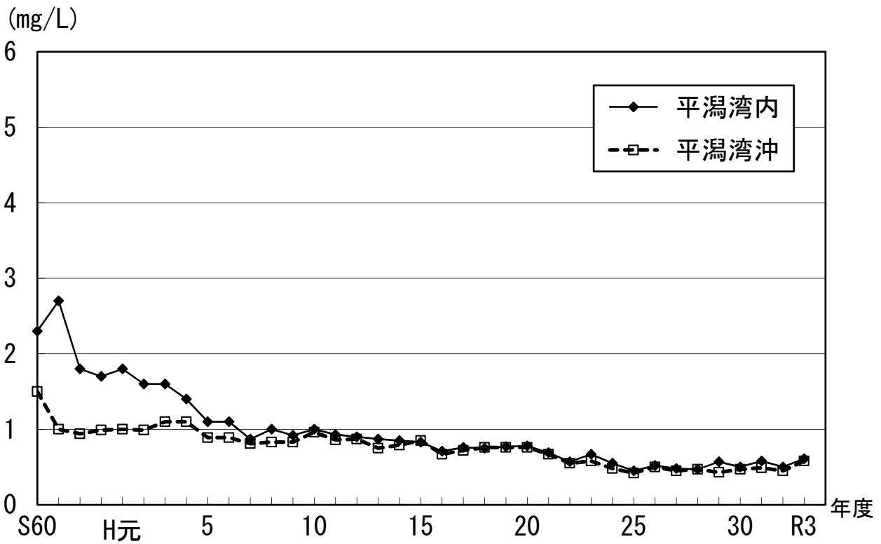
図 2-12 東京湾III類型全窒素年平均値の経年変化
