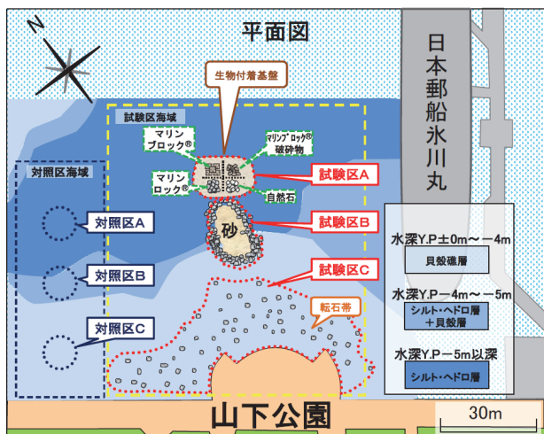
図 2 平面図
