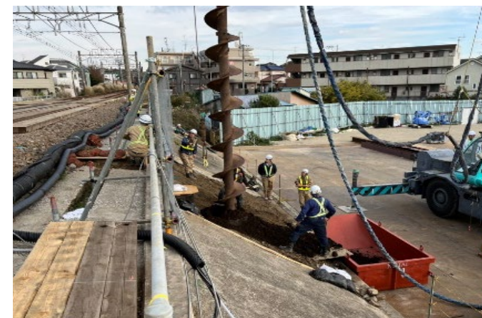
【相鉄線の土留め杭の工事の状況】
