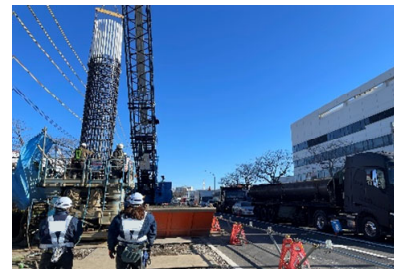
【橋りょう基礎杭の施工状況】
