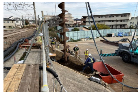
【相鉄線の土留め杭の工事の状況】
