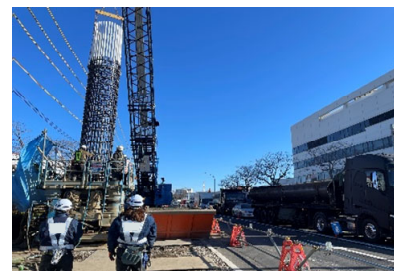
【橋りょう基礎杭の施工状況】
