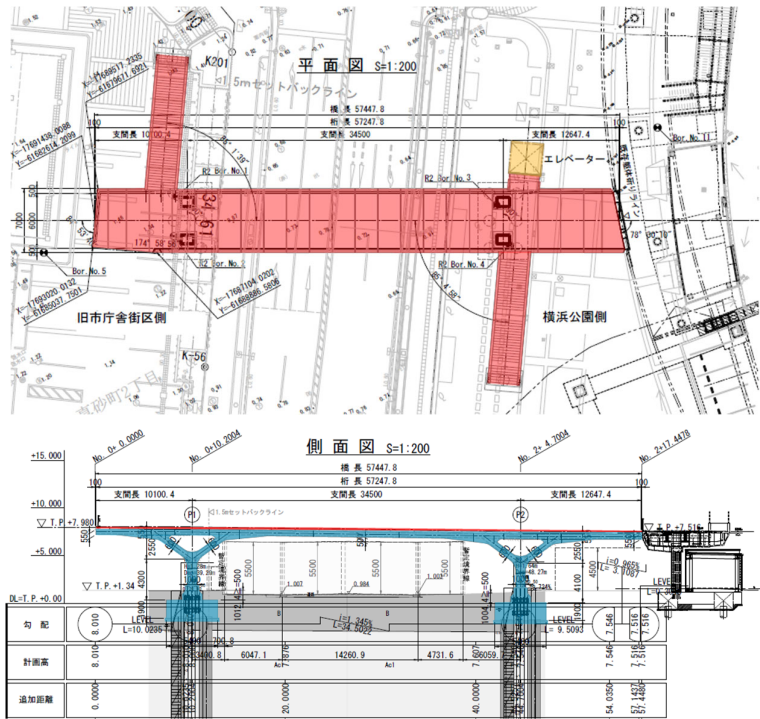
施設平面図・側面図・断面図
