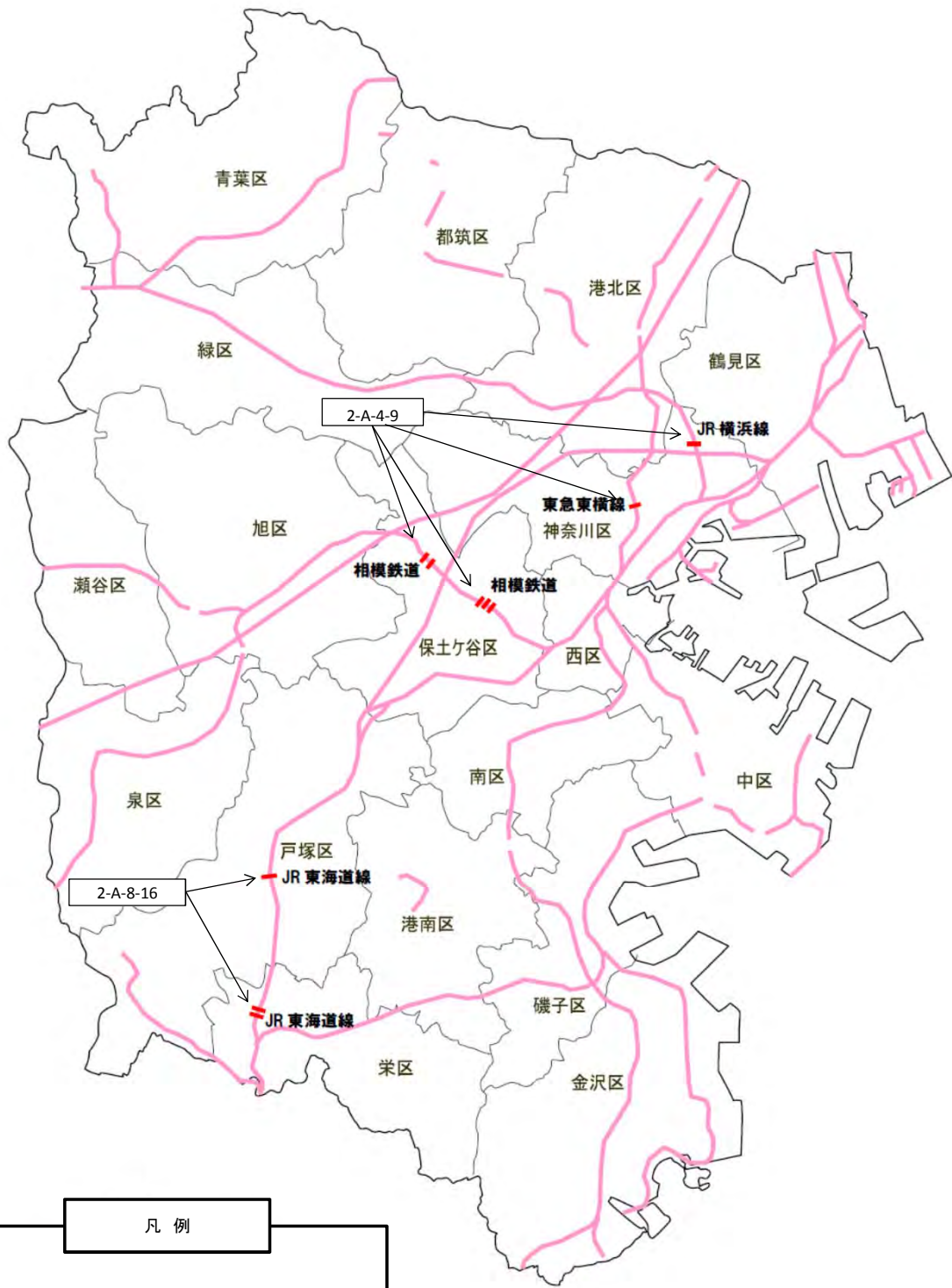
管きよの耐震化計画図(軌道下)
