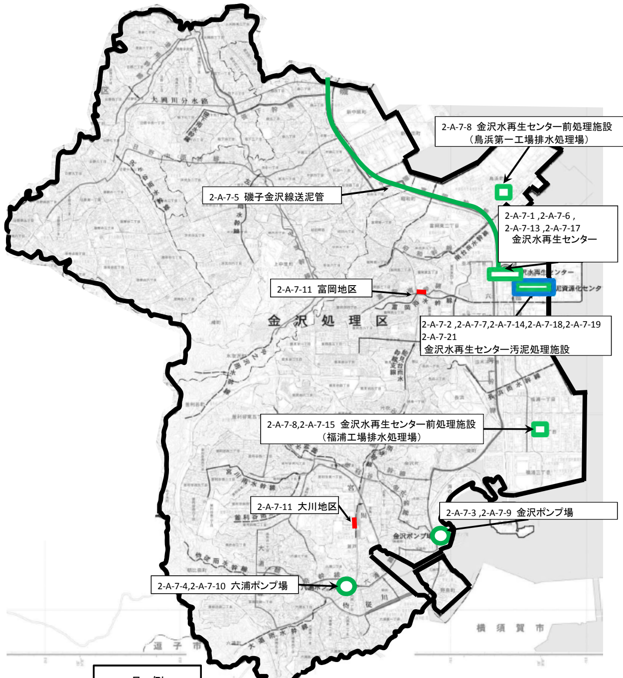
2-A-7,2-C-7 金沢処理区計画図
