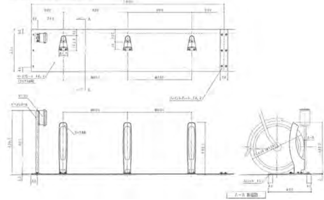
サイクルポート標準規格図
