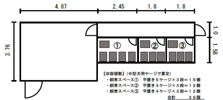
ペット避難所（飼育小屋）ケージ配置図
