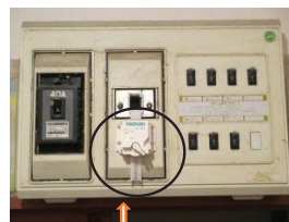
感震ブレーカー 標準取付の例
