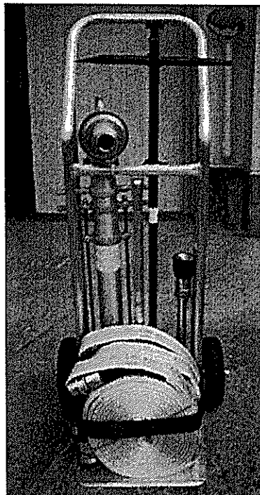
スタンドパイプ式初期消火用具
