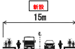
瀬谷地内線の新設
